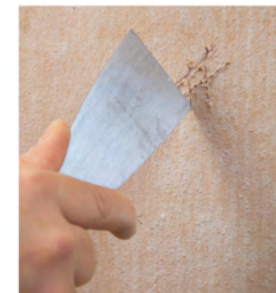
Kratzprobe Prüfen der Oberflächenfestigkeit
